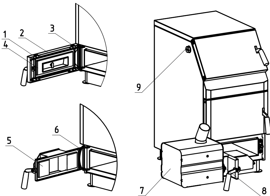
Рис. 7 Порядок установки двери на твердотопливные котлы ZOTA Тополь-М и ZOTA Master
