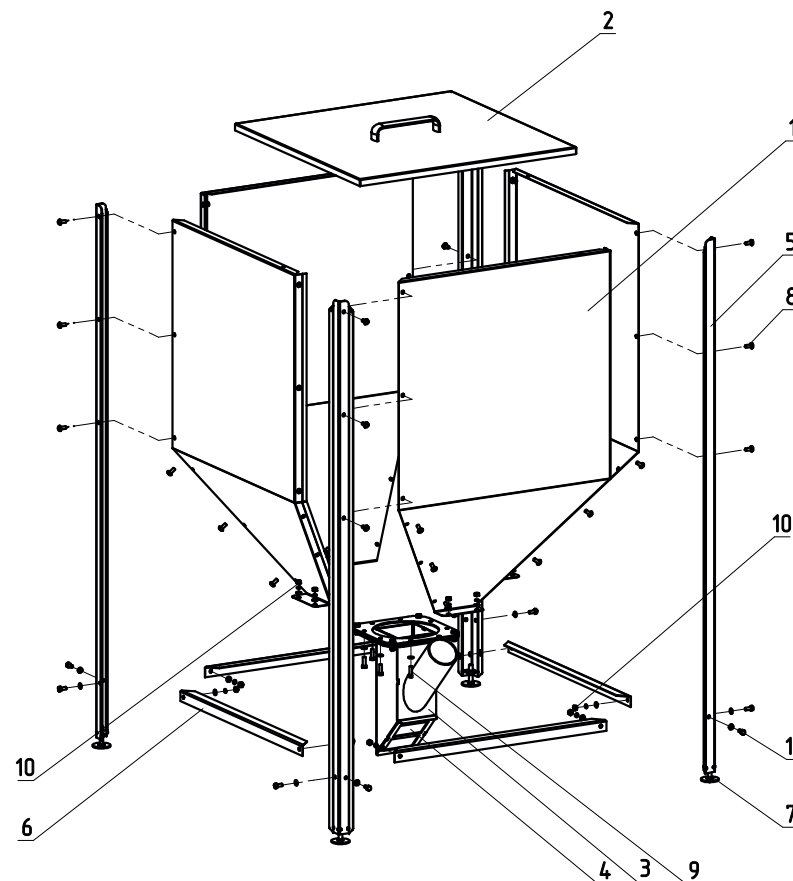
Рис.6 Порядок сборки топливного бункера
