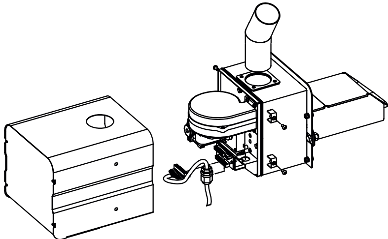
Рис. 10 Подключение кабеля управления к приставной пеллетной горелке
