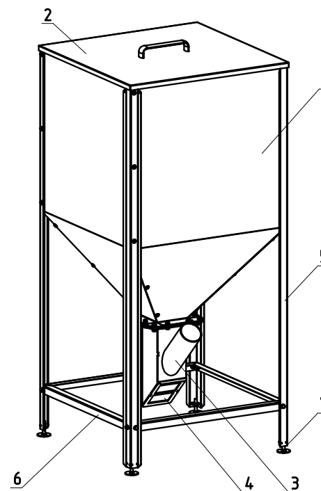
Рис.4 Топливный бункер
