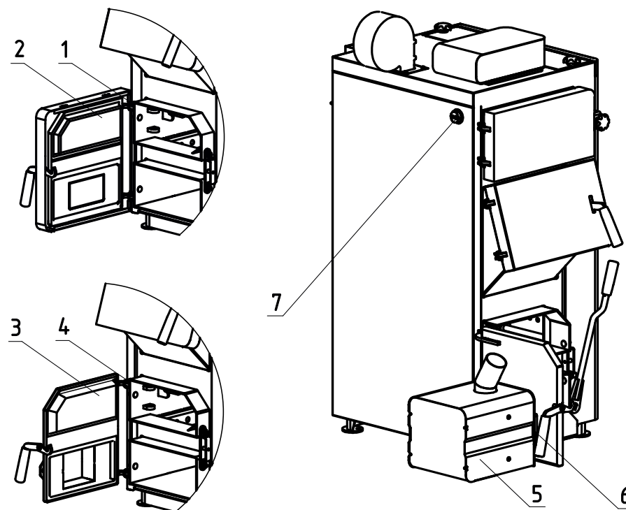
Рис. 10 Порядок установки двери на твердотопливные котлы ZOTA Magna 15;20;26
