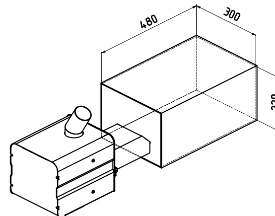
Рис. 11 Минимальные габариты топки котла
