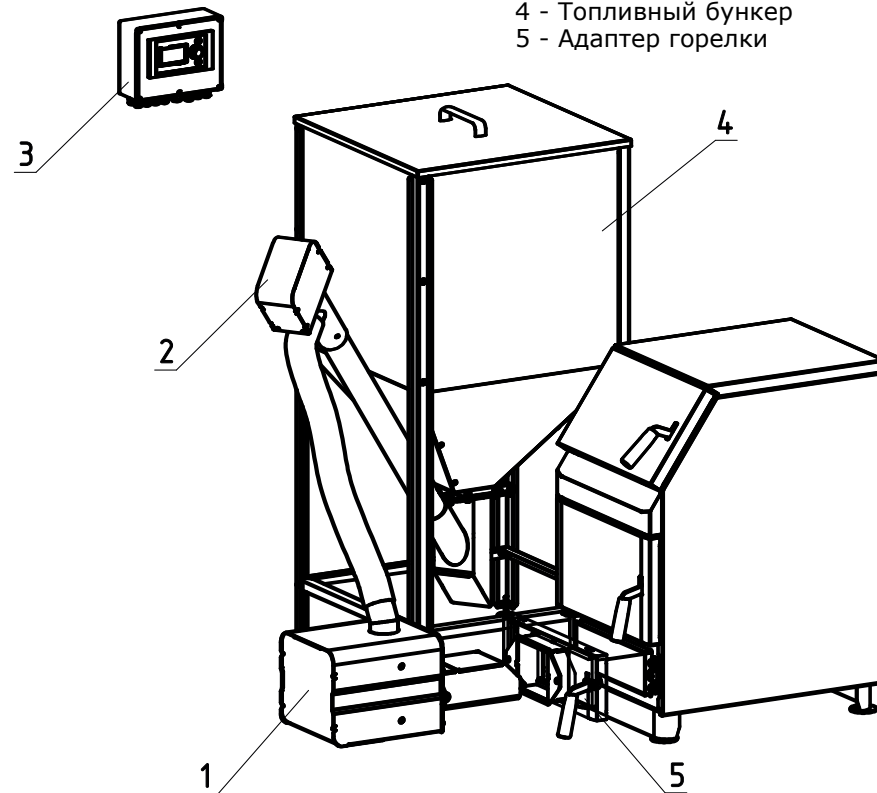
Рис. 1 Комплект приставной пеллетной горелки ZOTA Fox
